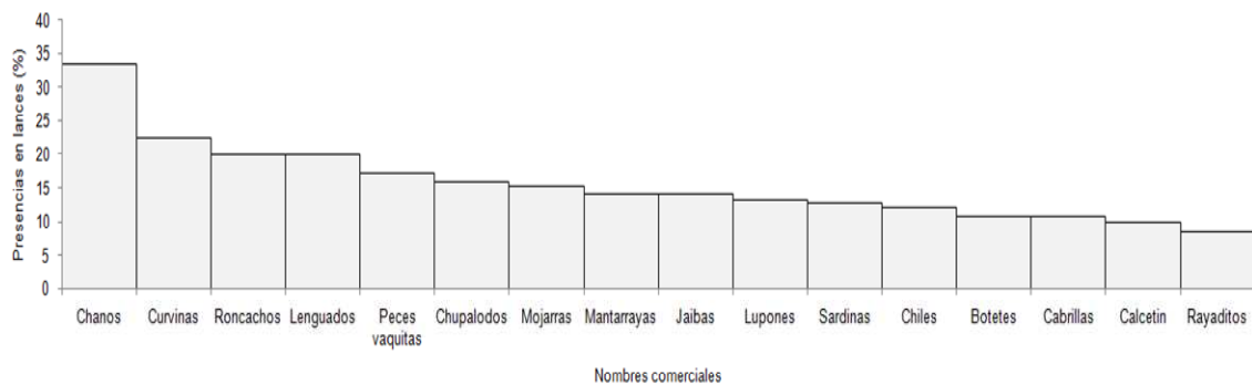
Figura 6. Porcentajes de las presencias o éxito en los lances realizados con red de arrastre, para las categorías de especies del elenco taxonómico que contribuyen con el 95% de las abundancias numéricas. En la parte superior se muestran los resultados de San Felipe BCS y en la parte inferior los resultados del golfo de Santa Clara Sonora durante 2010.
